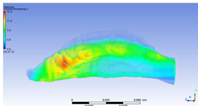
Рис. 2.5. Поле значений скорости течения воздуха в момент времени t = 1 (сценарий 25 °C) в носовой полости
