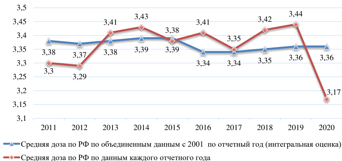
Рис. 1.105. Динамика средних индивидуальных годовых эффективных доз облучения населения Российской Федерации за счет природных ИИИ за период с 2011 по 2020 год, мЗв/год
